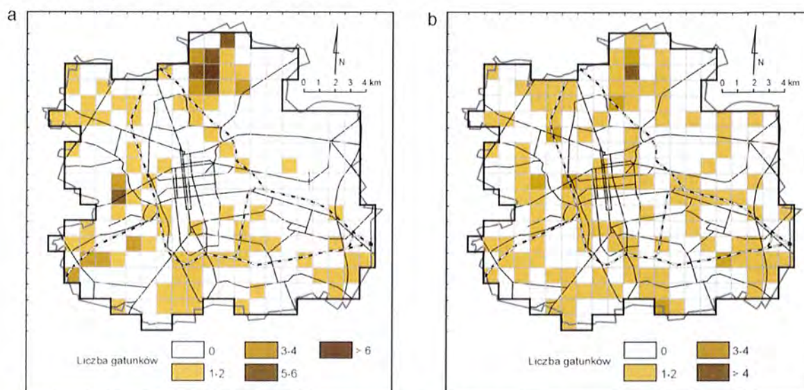
Rysunek 11 Przestrzenne zróżnicowanie zagęszczenia gatunków chronionych (a) i zagrożonych sensu stricto (b) 43
