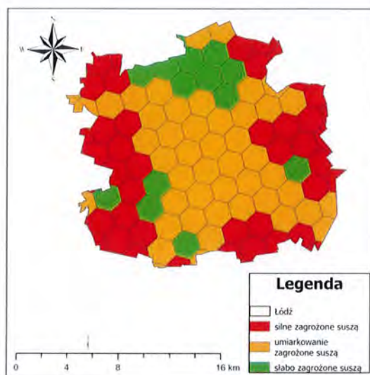
Rysunek 5 Łączne zagrożenie suszą na terenie Łodzi
