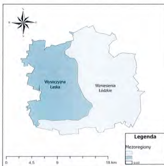
Rysunek 1 Mezoregiony fizycznogeograficzne na terenie Łodzi
