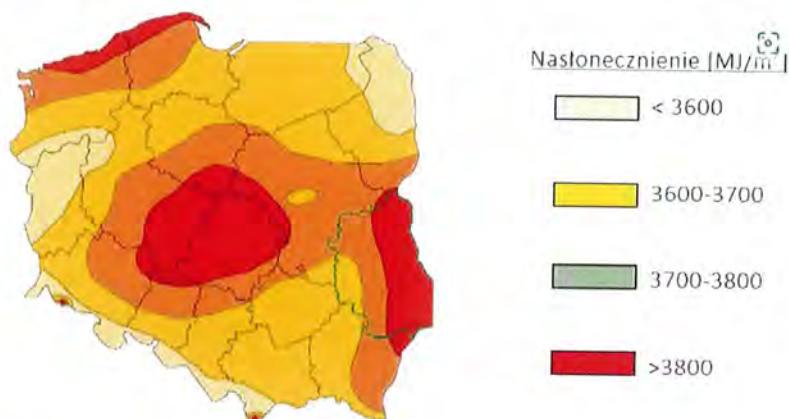
Rysunek 2 Nasłonecznienie w Polsce 9
