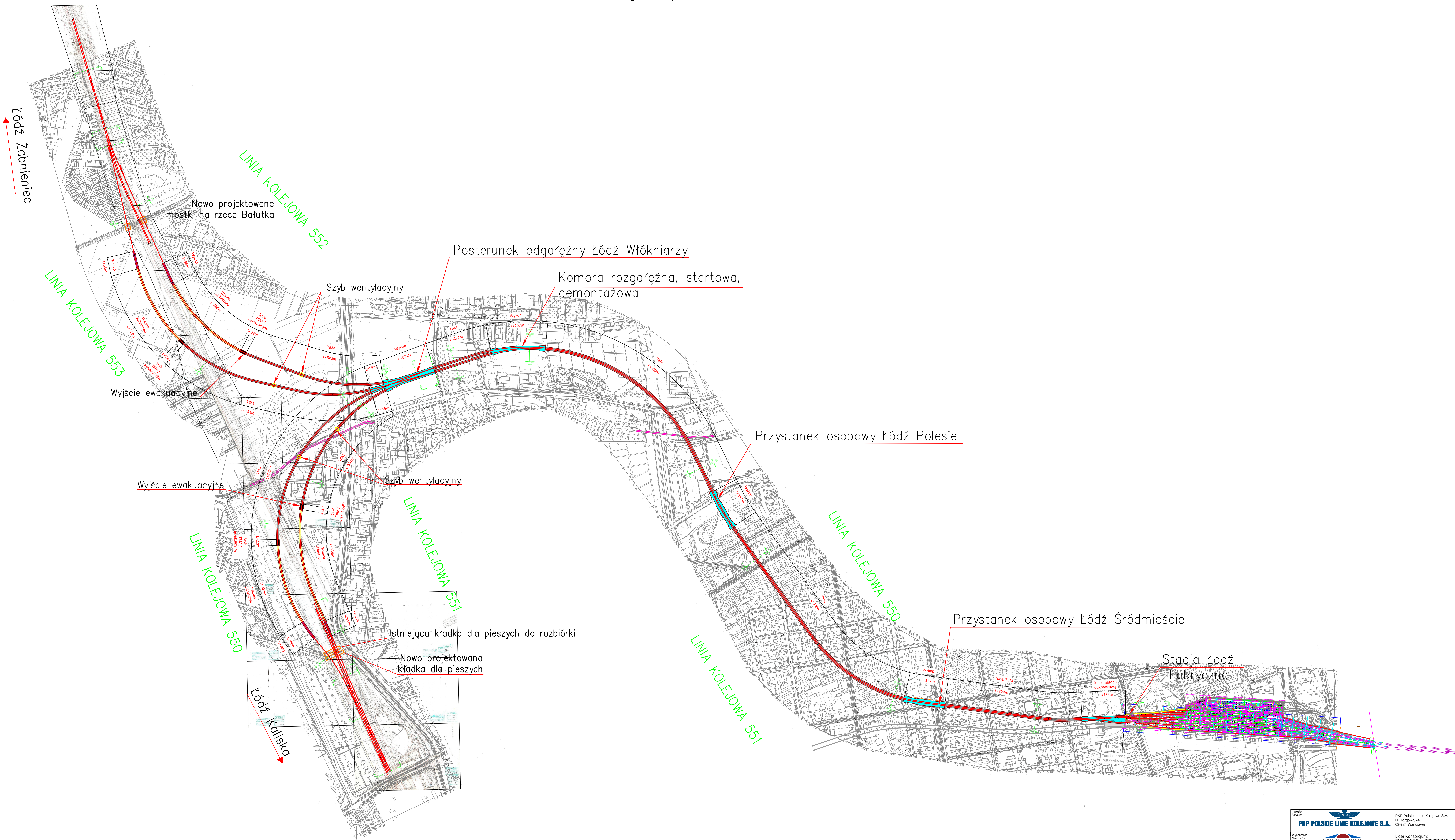
Widok trasy w planie skala 1:5000
