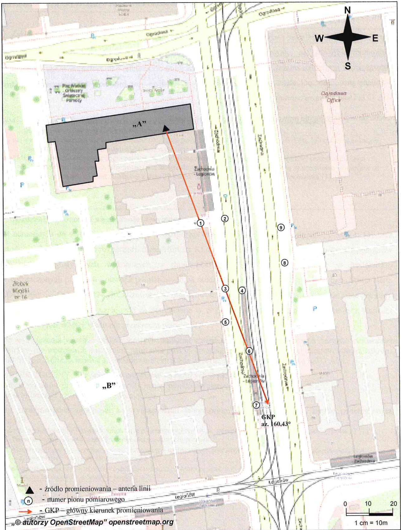
Rys. 1. Usytuowanie punktów i pionów pomiarowych w otoczeniu instalacji radiokomunikacyjnej Stacja Netia LODZD606-LODZM00474 Łódź, ul. Ogrodowa 16
